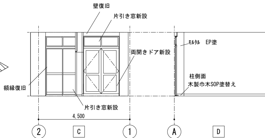
改修後展開図 1/100
