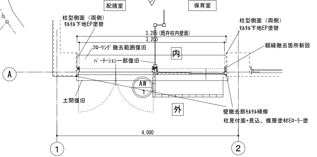
改修後平面詳細図 1/50
