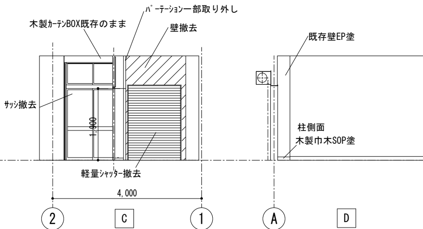
改修前展開図 1/100
