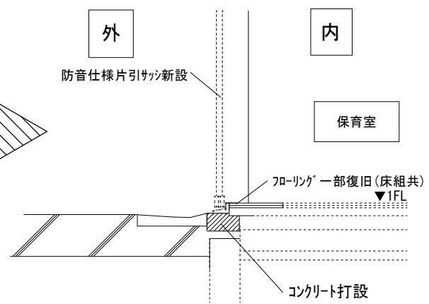
改修後保育室サッシ部断面図 1/30
