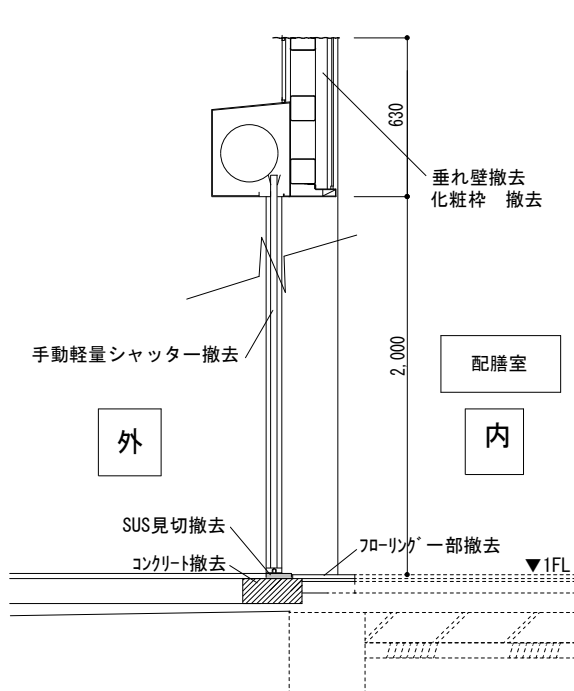
改修前配膳室側サッシ部断面図 1/30
