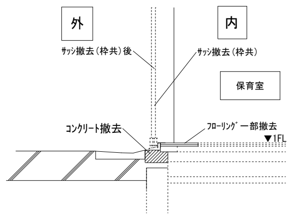
改修前保育室サッシ部断面図 1/30
