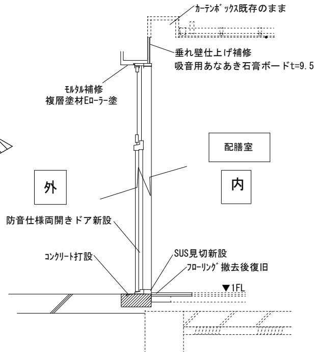
改修後配膳室側サッシ部断面図 1/30
