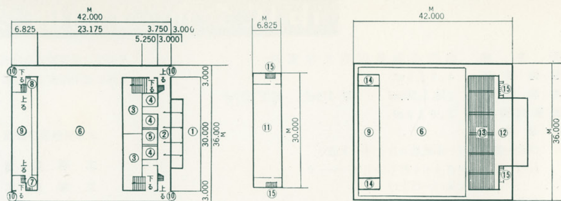
2階平面図
