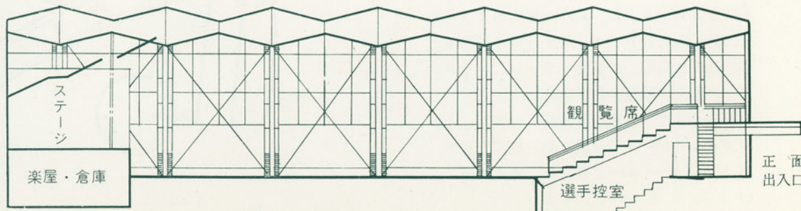
断面図
