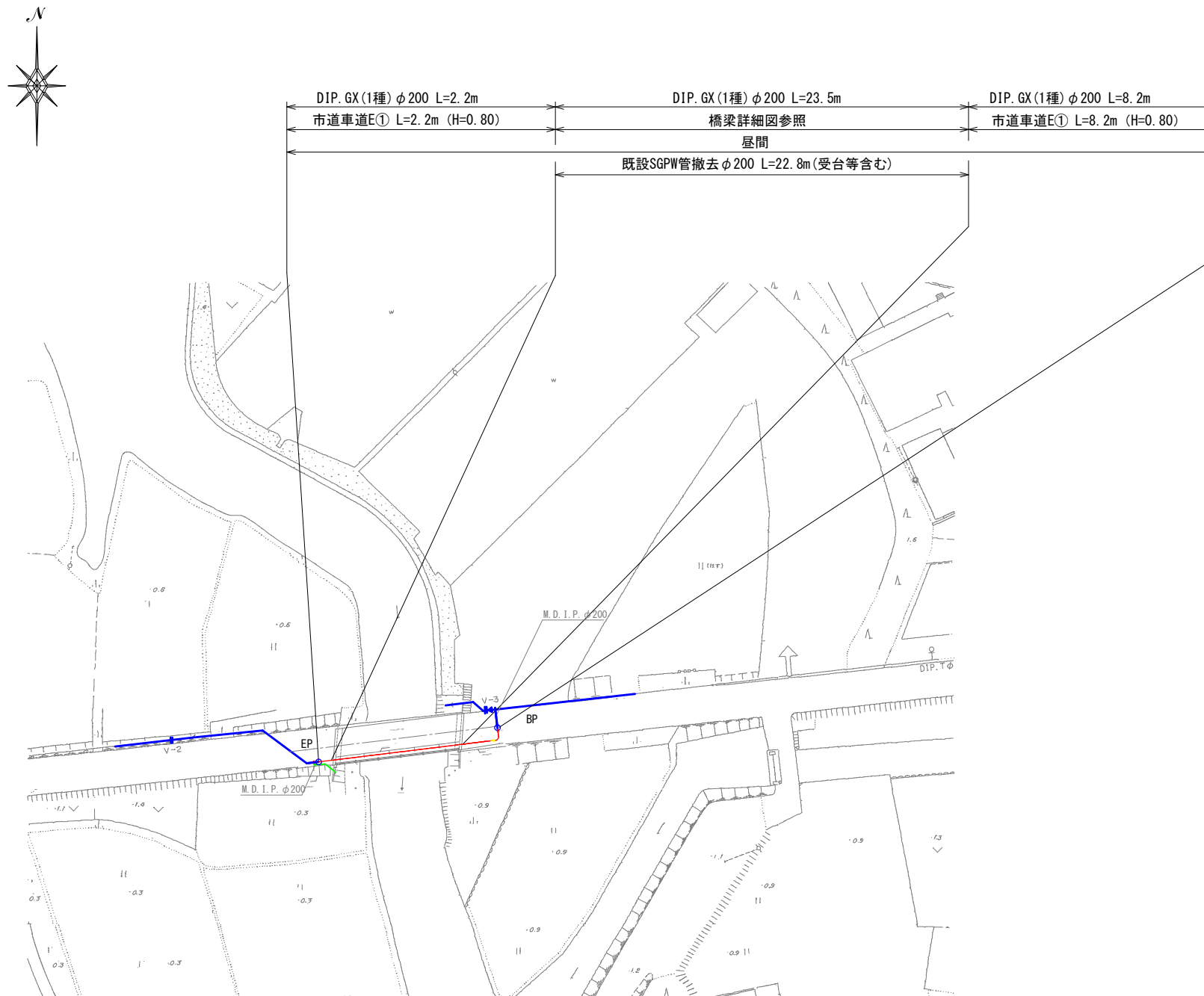
平面图 S=1:500
