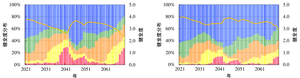
図 3.1 橋梁全体の評価指標（耐荷性）分布の推移：健全 危険
