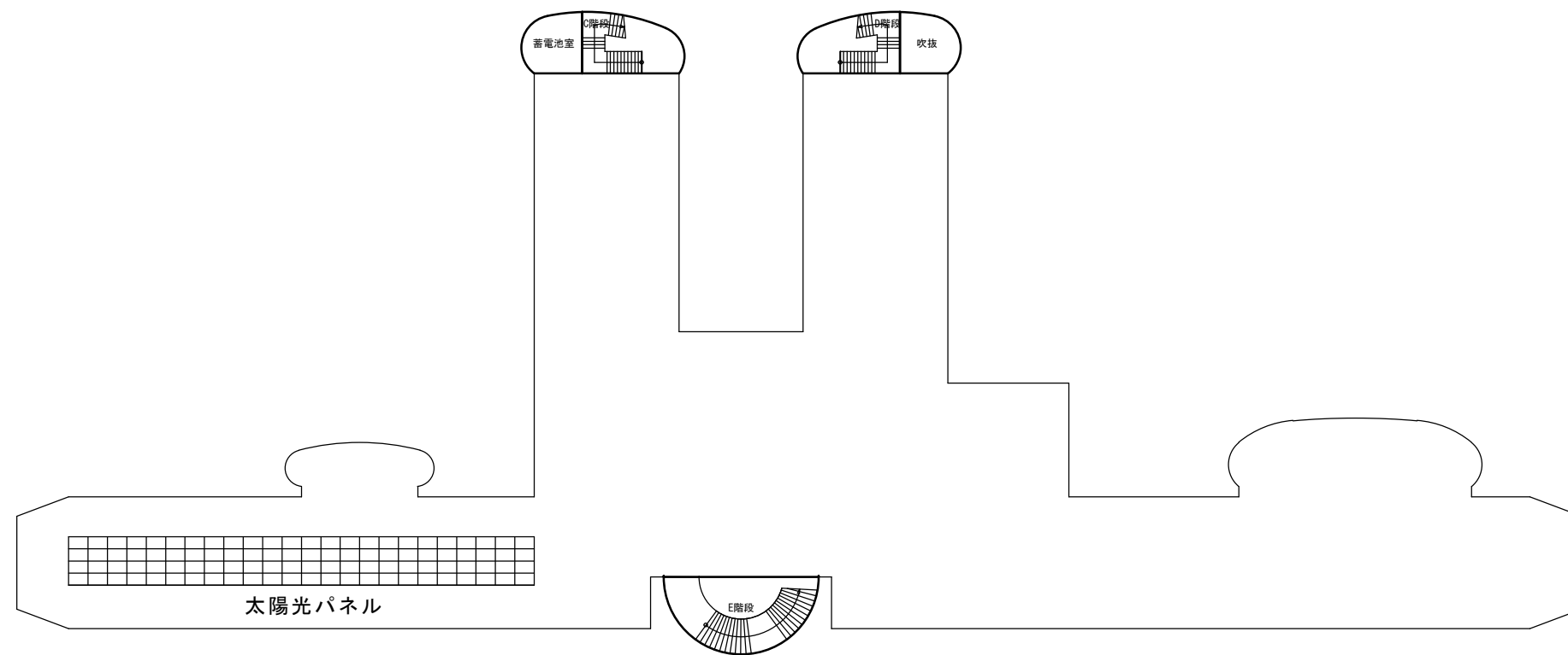
屋上平面図
