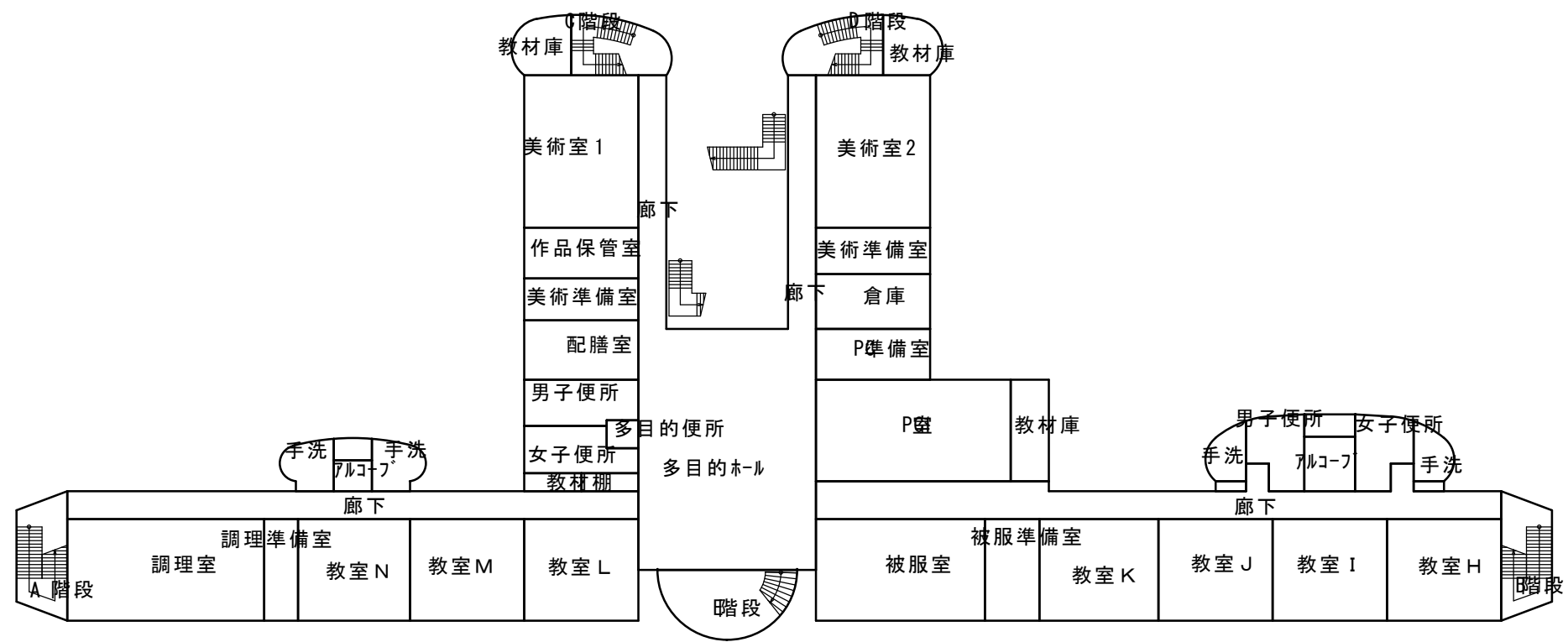
3 階平面図
